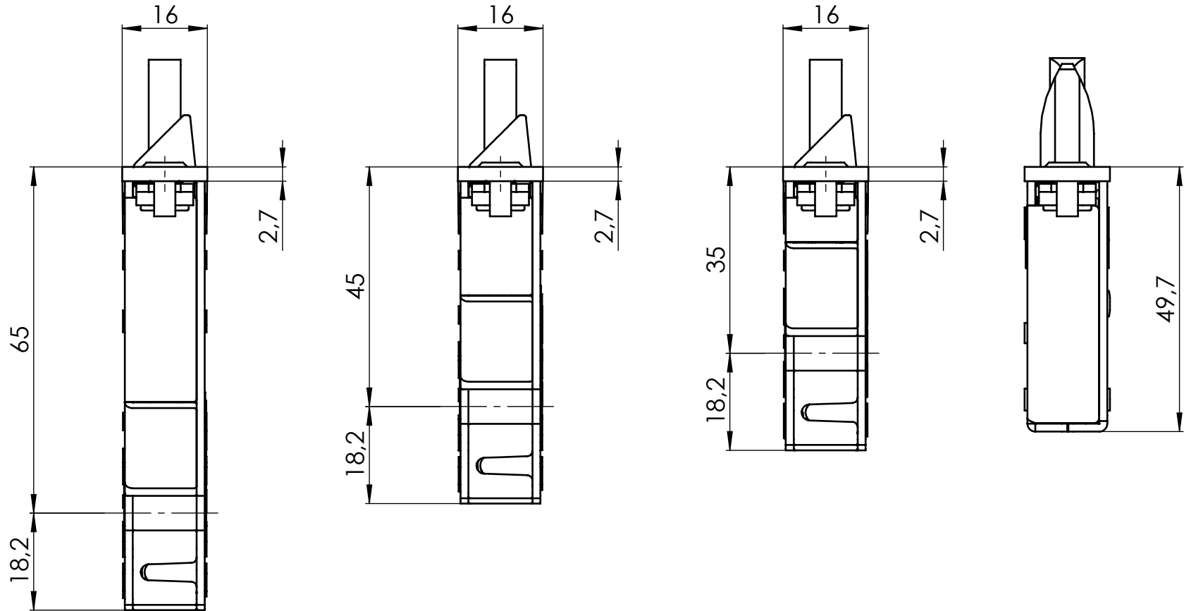
Ansicht in Pfeilrichtung A M 1:1
